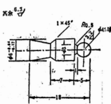
图 12.0.2-2 收缩头 (mm)
