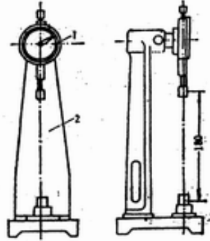
图 12.0.2-1 收缩仪 (mm) 1—千分表 2—支架
