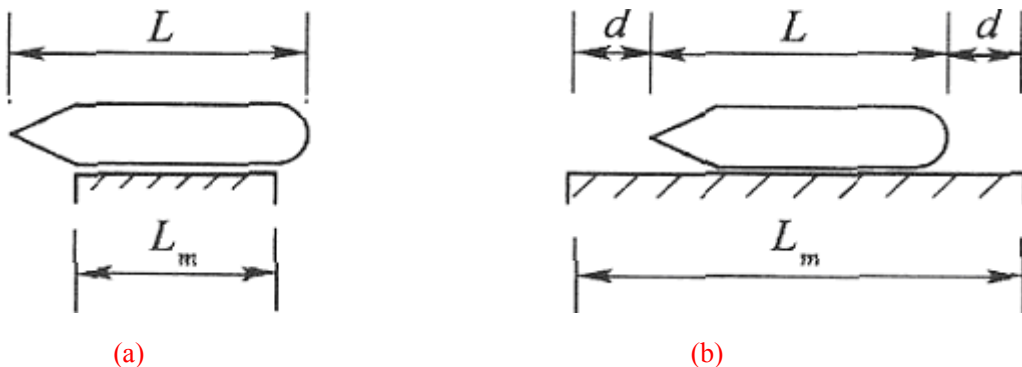
图 3.3.6.1 单个泊位的码头长度示意图((a)停靠内河驳；(b)停靠江海轮)
