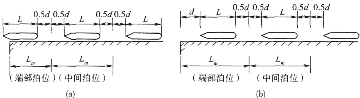
图 3.3.6-2 多个连续泊位的码头长度示意图
