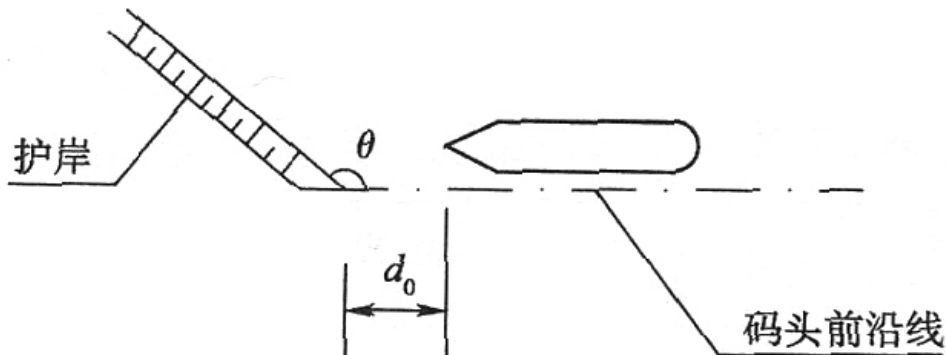
图 3.3.3-2 码头前沿线与护岸相交时富裕长度示意图
