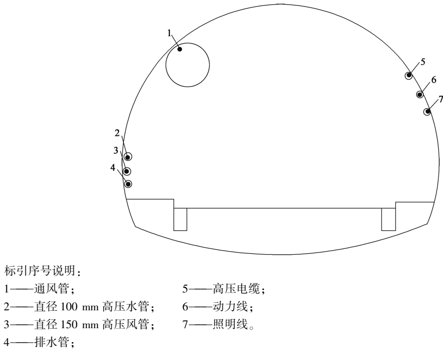
图 5 洞内隧道线路布设示意图
